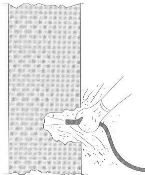
Figura 10.4 – Exemplo de procedimento de Jateamento de Ar Comprimido.
