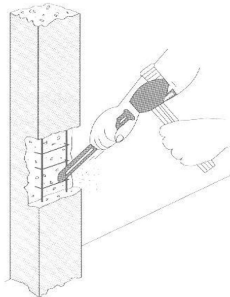
Figura 10.1 – Exemplo de procedimento de escarificação meramente ilustrativo.
