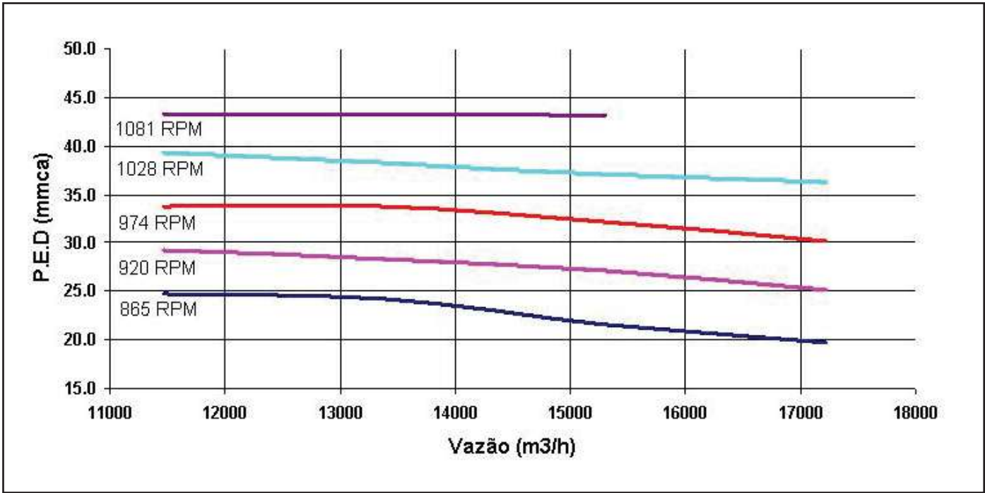
Curvas de Vazão de Ar 40B 25 Heavy VH
